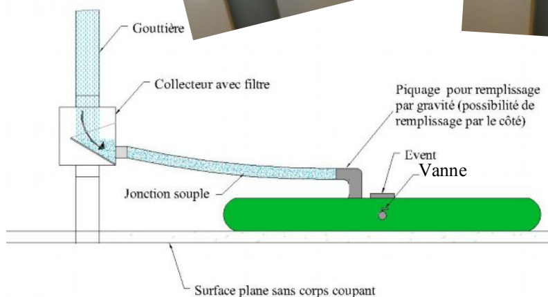
CITERNE EN COURS DE REMPLISSAGE
